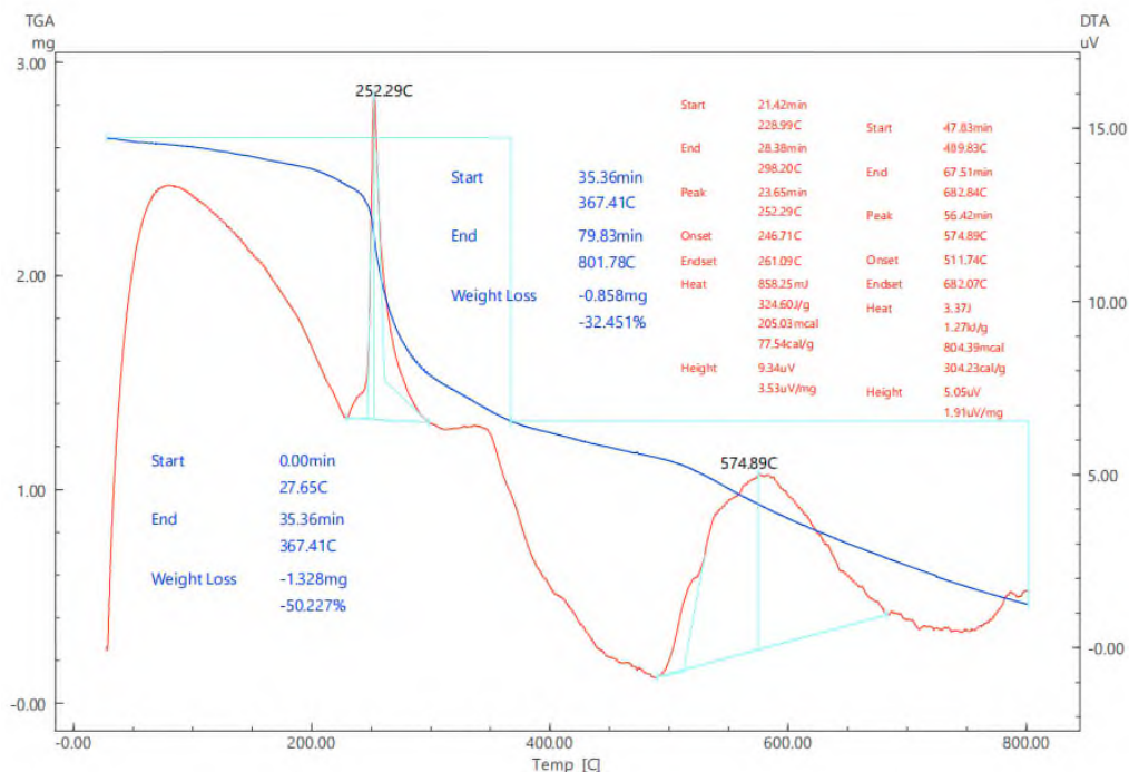
2-rasm. \text{H}_2\text{L} asosida olingan \text{CuL}\cdot\text{NH}_3 kompleksining TGT, DTT, DSC grafiklari.
