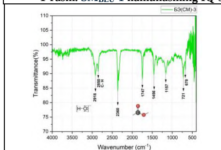
3-rasm. SM BEU -3 namunasining IQ-spektri.
