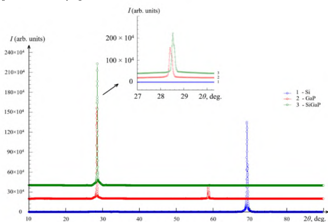
3-rasm. Fosfor va galliy kirishma atomlari bilan legirlangan kremniyning rentgenogrammasi va rentgenogrammaning kattalashtirilgan shkalasi.
