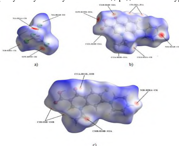
3-расм. [\text{CdCl}_4]^{2-} -анион ва (\text{HL})^+ -катионлари учун уч ўлчамли Хиршфельд юзасининг тасвири -0,4180 дан 1,3344 гача бўлган диапазонда d_{\text{норм}} бўйлаб чизилган (Бу ерда, а [\text{CdCl}_4]^{2-} -анион учун, (b) ва (c) мос равишда \text{ClP(A)}^+ ва \text{ClP(B)}^+ катионлари учун Хиршфельд юзаларидир).
