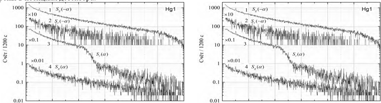
Рис. 2. Спектры сформированных S_g(-\alpha) – 1 и S_g(\alpha) – 4 и рефлекторных S_r(\alpha) – 3 и S_r(-\alpha) – 2
