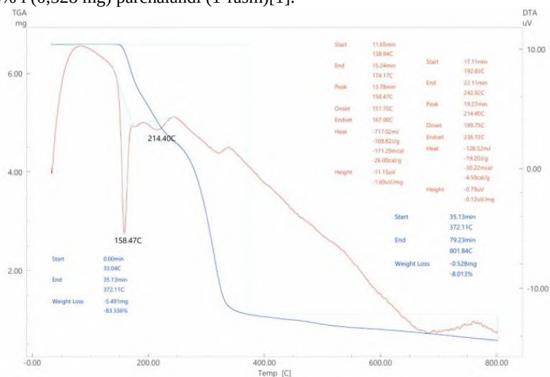
2-rasm. H_2L ning TGT, DTT, DSC grafiklari.
