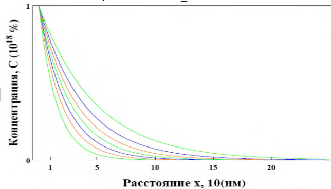
Рис. 2. Зависимость концентрации кислорода от глубины кремниевой пластины.
