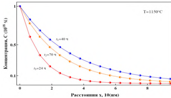
Рис. 1. Профиль концентрации кислорода.
