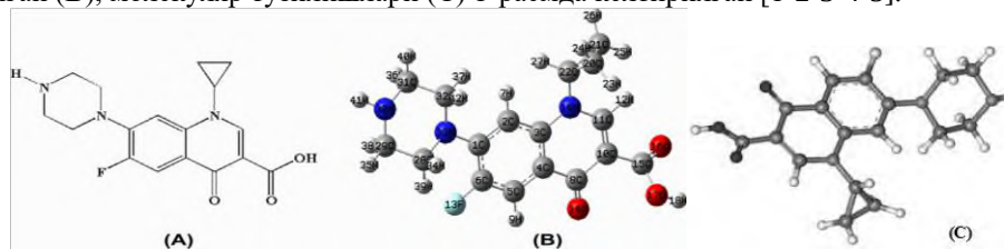
1-расм. Ципрофлоксациннинг кимёвий (A) ва оптималлаштирилган (B) ва молекуляр тузилишлари (C)
