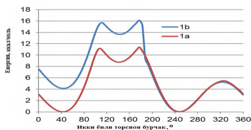
3-расм. Ципрофлоксацин (1a) ва унинг протонланган (1b) ҳолатлари мисолида циклопропан ҳалқасининг ички айланиш потенциал сатҳи эгри чизиқлари
