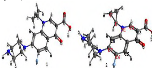
2-расм. Фазовий жихатдан бир-бирдан фарқ қилувчи 1 ва 2 ципрофлоксацин молекулаларининг DFT усулида мақбуллаштирилган фазовий тузилиши (C2-N1-C-C ва C6-C7-N-C торсион бурчаклар мос равишда циклопропан ҳамда пиперазин ҳалқаларини C-N боғи атрофида айлантириш учун қўлланилди).
