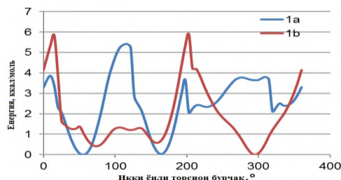
3-расм. Ципрофлоксацин (1a) ва унинг протонланган (1b) ҳолатлари мисолида пиперазин ҳалқасининг ички айланиш потенциал сатҳи эгри чизиқлари
