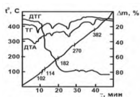
Рисунок 3. Дериватогрмма комплексной соли \text{NH}_2\text{C}_2\text{H}_4\text{OH} (\text{CH}_3\text{COO})_2\text{Cu} \cdot \text{H}_2\text{O} состава 1:1
