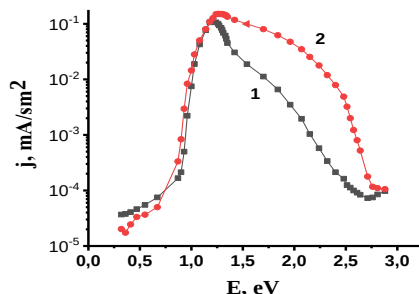
2-rasm. Fosfor kirishma atomlari bilan (1) va galliy va fosfor kirishma atomlari bilan (2) legirlangan kremniyning fotoelektrik xossalari
