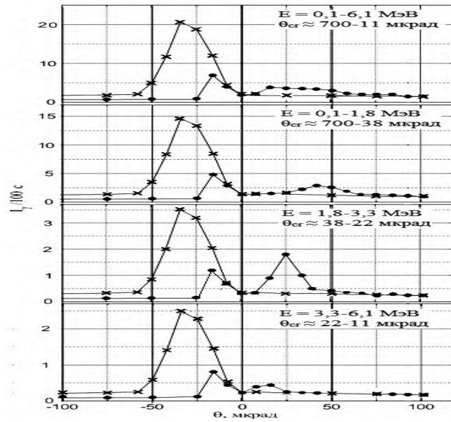
Рис 3. Угловые распределения гамма-квантов сформированного (×) и рефлекторного (•) пучков ТИЭ в различных энергетических диапазонах с рефлектором Hg2.
