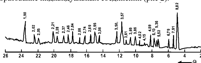
Рисунок 2. Рентгенограмма соединения моногидрата ацетата меди с моноэтаноламином при соотношении моногидрат ацетат меди:моноэтаноламин 1:1
