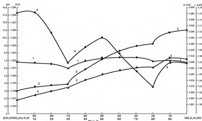
Рисунок 1. Система моногидрат ацетата меди – моноэтанолламин – вода: 1 – показатель преломления, 2 – pH-среды, 3 – плотность, 4 – вязкость
