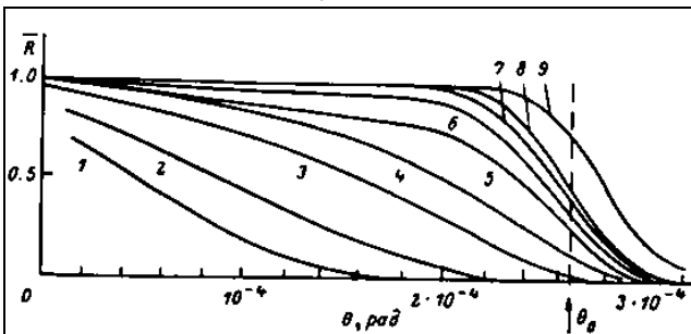
Рис 8. Зависимость R(9) для пучков с расходимостью 6 \times 10^{-6} \text{ рад} . \alpha/h_p=1000 (1) , 500 (2) ,200 (3), 100 (4) , 50 (5), 20 (6), 10 (7), 5 (8), 0 (9).
