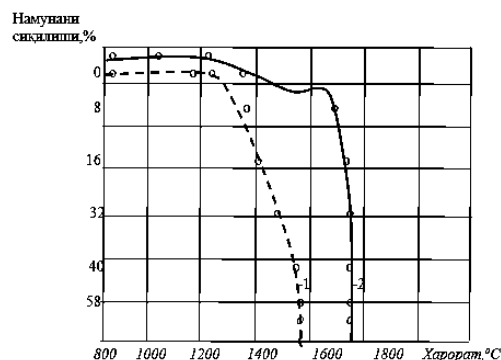
3-расм. Намунага бир вақтнинг ўзида юқори харорат ва зарбали тўлқин (сиқилиш кучланиши) таъсир эттирганда деформацияга бардошлик кўрсаткичлари: 1- саноат бетон намунаси, 2-“МНА”-русумидаги полимер қўшилган асбестоцемент билан қопланган бетон намунаси.
