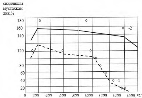
2-расм. Тажриба-синов намуналарининг юқори харорат таъсирида сиқилишга мустахкамлиги кўрсаткичининг ўзгариш динамикаси: 1- саноат бетон намунаси, 2- “МНА”-русумидаги полимер қўшилган асбестоцемент билан қопланган бетон намунаси.
