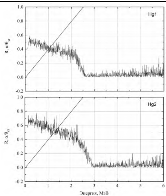
Рис. 5. Энергетические зависимости коэффициента отражения пучков ТИЭ от рефлекторов Hg1 и Hg2 ( \alpha = 30 мкрад)
