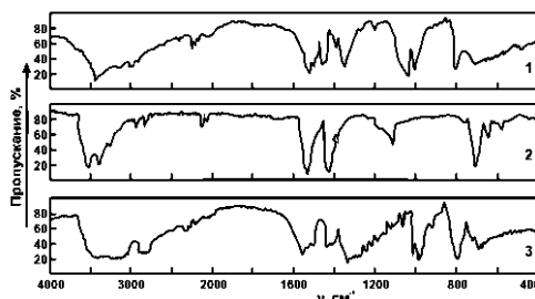
Рисунок 4. ИК-спектры: 1-моноэтаноламин, 2-моногидрат ацетат меди, 3-соединение состава в соотношении 1:1
