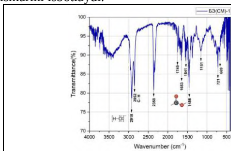
1-rasm. SM BEU -1 namunasining IQ-spektri.
