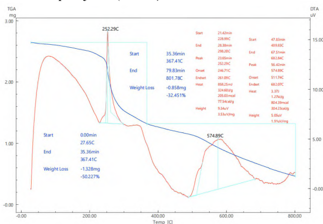
2-rasm. H_2L asosida olingan CuL \cdot NH_3 kompleksining TGT, DTT, DSC grafiklari.
