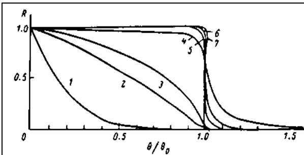
Рис7. Зависимость коэффициента отражения R(6) для пучка с нулевой расходимостью от угла скольжения \theta .
