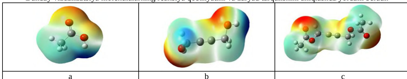
5-Rasm.a) metan kislota b) butin-2-diol-1,4 c) butin-2-diol-1,4 diformiat strukturalarining optimallashtirilgan ESP natijalari ESP tahlili
