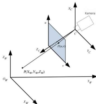
4-rasm. Kameraning chiziqli tasvirlash modeli.
