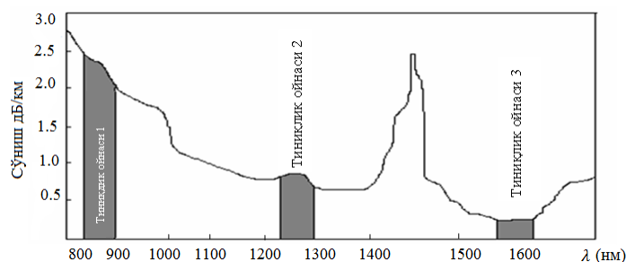
7-расм. Тўлқин узунлигига боғлиқ равишда оптик тола сўнишининг ўзгариши.
