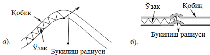
5-расм. Оптик толанинг макробукилишлари (а) ва микробукилишлари (б).
