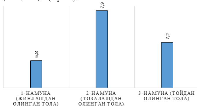
1-расм. Калта толалар индекси (SFI) нинг ўзгариши
