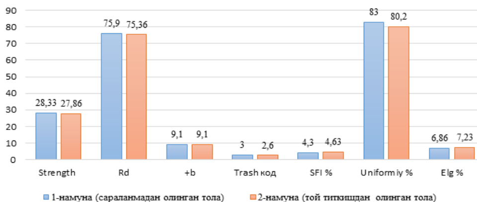
3-расм. Тола хоссаларининг титиш жараёнида ўзгариши
