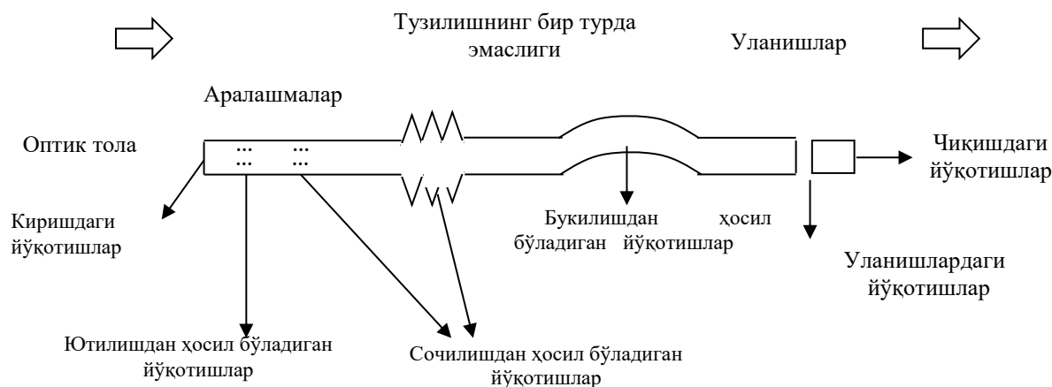
6-расм. Оптик сигнални узатиш сифатига таъсир қилувчи омиллар.
