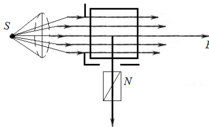
2-расм. Хира муҳитларда ёруғлик сочилишини кузатиш схемаси.
