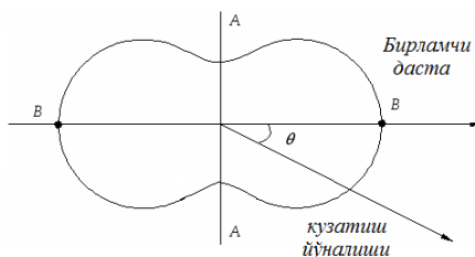
3-расм. \lambda га нисбатан кичик бўлган зарралар учун сочилиш индикатрисаси.
