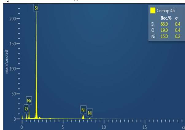
Рис. 2. Состав кластеров примесных атомов никеля «Спектр 46» определенный с использованием метода энергодисперсионной рентгеновской спектроскопии EDS.
