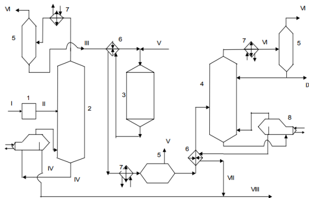
2-súwret. UNTDU tárepinen islep shıǵılǵan Rigiz procesiniń ulıwma texnologiyalıq sxeması: 1-riforming apparatı; 2-rektifikaciya kolonnası; 3-gidrlew reaktori; 4-turaqlılastırıw kolonnası; 5-gazoseparator; 6-ıssılıq almastırǵısh; 7-suwıtqısh; 8-riboylar. I aydalǵan shiyki zat; II riformat; III riformingnıń jenil frakciyası; IV riformingnıń qaldıq frakciyası; V vodorod saqlaǵan gaz; VI ulevodorodlı gaz; VII turaqlı gidrogenizat; VIII ekologiyalıq qásıyetleri jaqsılǵan joqarı oktanlı benzin komponenti; IX reflyuks.
