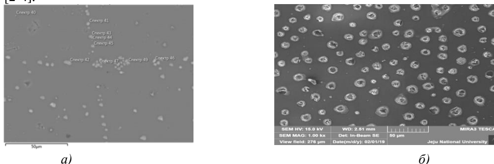
Рис. 1 Распределение кластеров на поверхности кремния полученное с помощью сканирующего электронного микроскопа MIRA 3 TESCAN, (Field-Emission Scanning Electron Microscope (FE-SEM))
