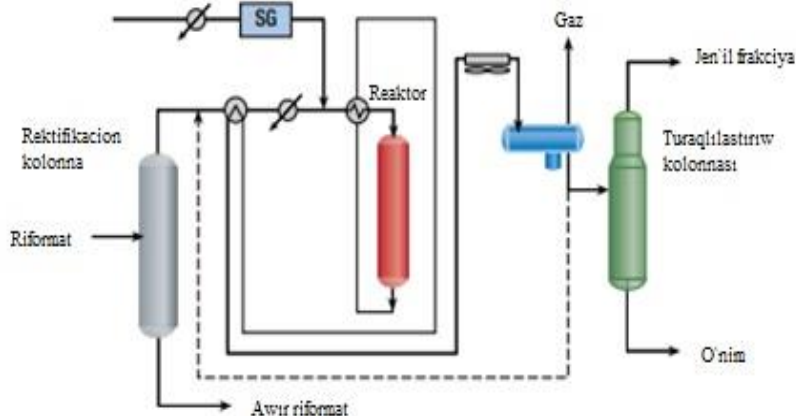
1-súwret. UOP firmasınıń Bensat apparatınıń texnologiyalıq sxeması
