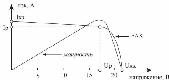
Рис.4. ВАХ согласно (4) и зависимость мощности (5) от величины фотоЭДС.
