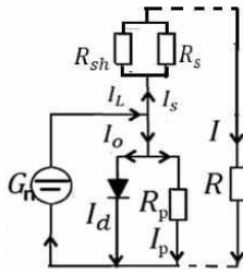
Рис.2. Эквивалентная схема солнечного элемента с наноразмерным гетеро переходом.
