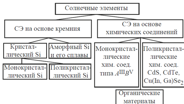
Рис1. Типы солнечных элементов
