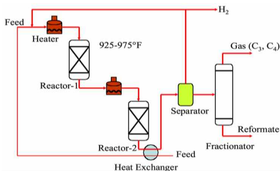
Рис. 1.1. Каталитический риформинг с непрерывной регенерацией катализатора
