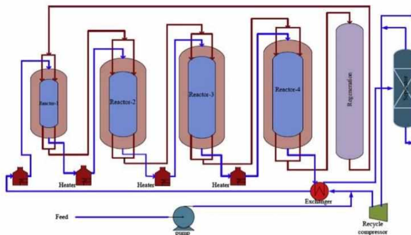
Рис. 1.2. Технологическая схема CCR процесса с расположением реакторов друг за другом: Feed – сырьё (нафта); Reactor 1,2,3,4 – реактор 1,2,3,4; Heater – нагреватель (печь); Recycle Compressor – компрессор; Regenerator – регенератор; Exchanger – теплообменный аппарат; Separator – сепаратор; Pump – насос.
