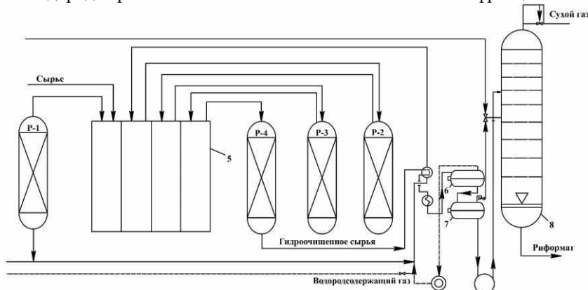
Рис. 1.4. Принципиальная схема установки риформинга бензинов с неподвижным слоем катализатора: P-1 – реактор гидроочистки; P-2, P-3, P-4 – реакторы риформинга; 5 – многосекционная печь; 6, 7 – сепараторы высокого и низкого давления; 8 – стабилизационная колонна.
