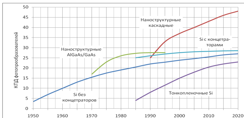
Рис. 2. Динамика увеличения КПД фотопреобразователей на основе кремния и наноструктур
