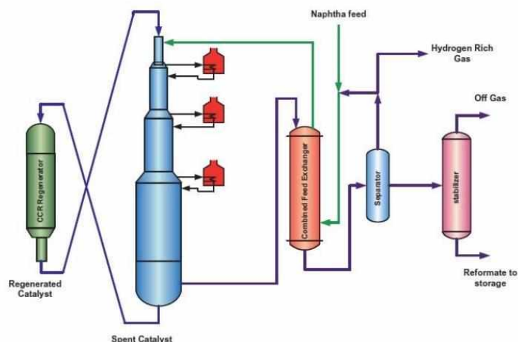
Рис. 1.3. Технологическая схема CCR процесса с расположением реакторов друг на друге: Naphtha feed – сырьё (нафта); Hydrogen Rich Gas – ВСГ; Off Gas – отработанный газ; Reformate to Storage – риформат; Regenerated Catalyst – регенерированный катализатор; Spent Catalyst – отработанный катализатор; CCR Regenerator – CCR регенератор; Combined Feed Exchanger – комбинированный сырьевой обменный аппарат; Separator – сепаратор; Stabilizer – стабилизатор.
