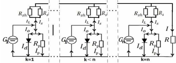
Рис.3. Эквивалентная схема солнечного элемента со многими наноразмерными гетеро переходами.
