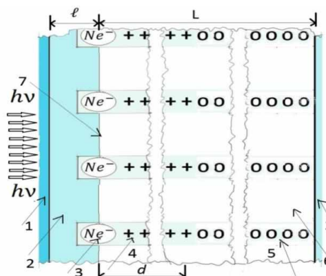
Рис.1. Модель солнечного элемента с наноразмерными p-n переходами.
