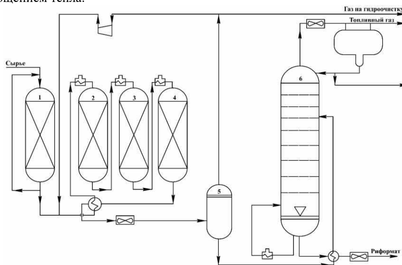
Рис. 1.5. Принципиальная схема установки риформинга по технологии компании Шеврон: 1 – реактор гидроочистки; 2, 3, 4 – реакторы риформинга; 5 – сепаратор; 6 – стабилизационная колонна
